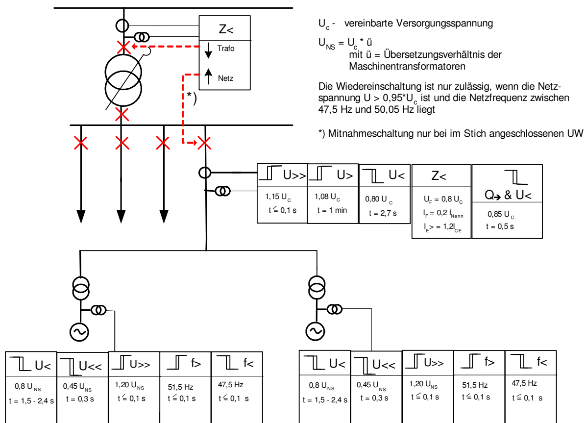
Bild 3.2.3.3-1: Schutzkonzept bei Anschluss von Erzeugungsanlagen an die Sammelschiene eines Umspannwerkes.
